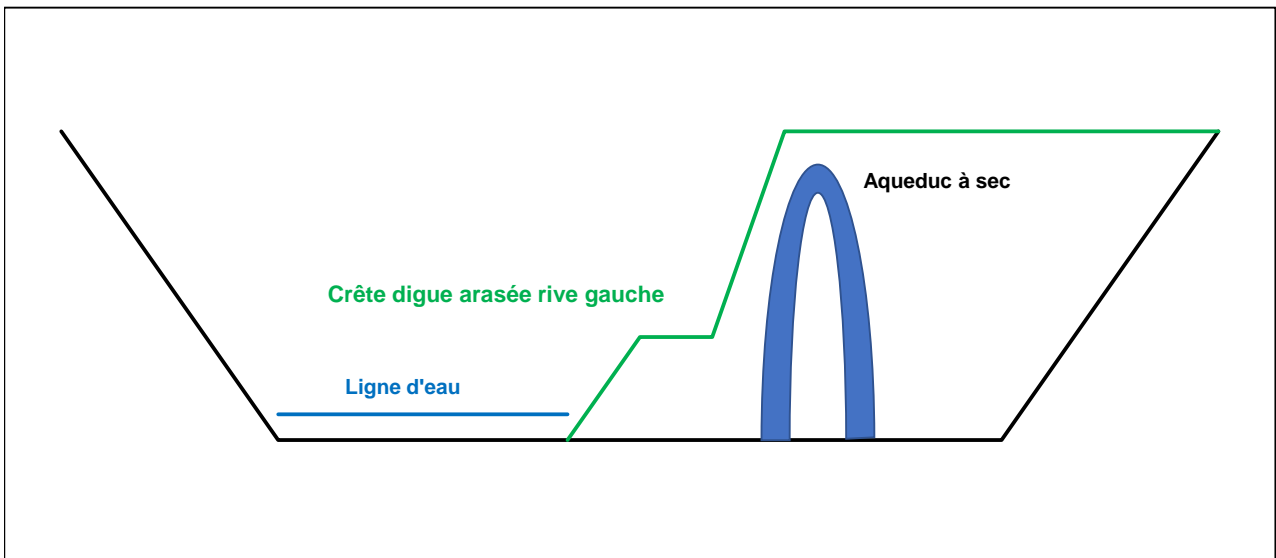
Situation intermédiaire avec ouverture totale de la digue en rive gauche pour travailler en assec total sur la rive droite
